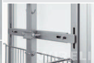
detal mocowania frontu przy pomocy ramy 3D
