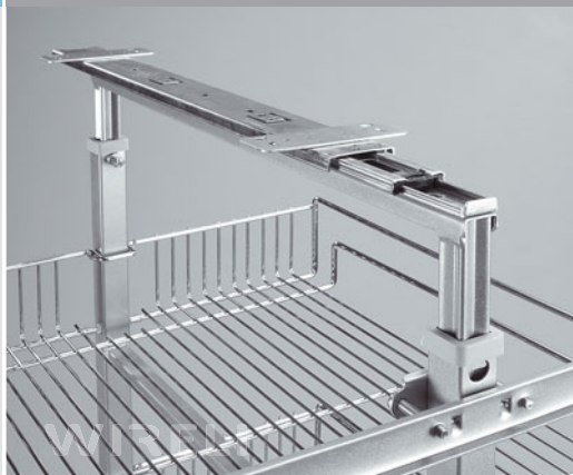
górną prowadnicę i mechanizm nastawienia wysokości ramy
