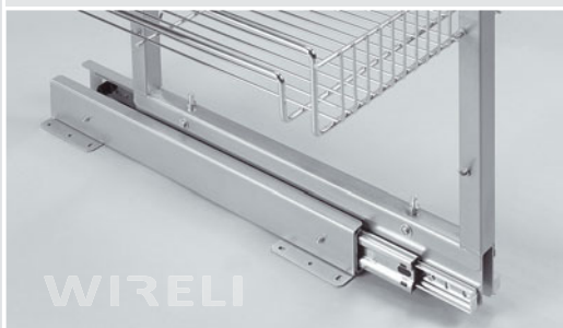
dolną prowadnicę z tłumionym domykaniem
