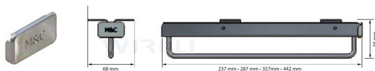
Zaślepka z logo
