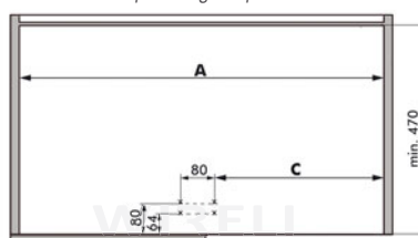
montaż do korpusu bez pionowego słupka
