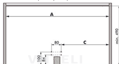
montaż do korpusu z pionowym słupkiem
