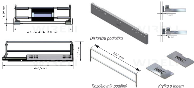
Rozdělovník podélný
