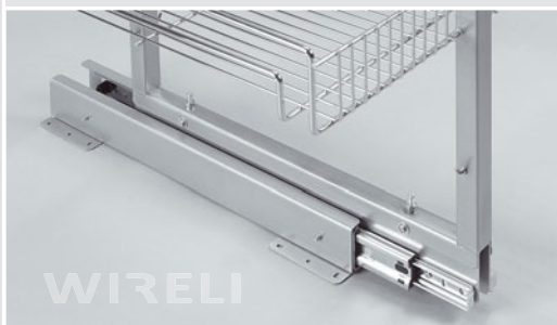
detail spodního výsuvu a uchycení rámu
