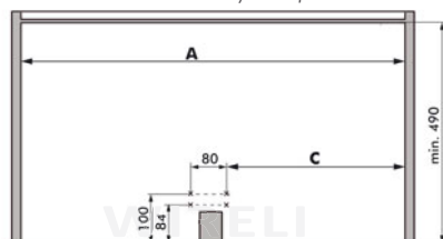
montáž do skřínky s vertikálním středovým sloupkem
