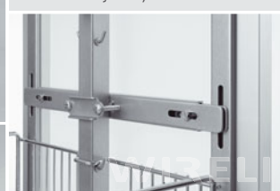
detail uchycení dvířek pomocí 3D stavitelného rámu
