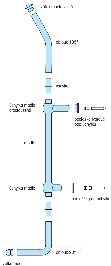
montáž závěsného systému
